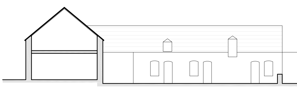
Bâtiment B façade ouest
